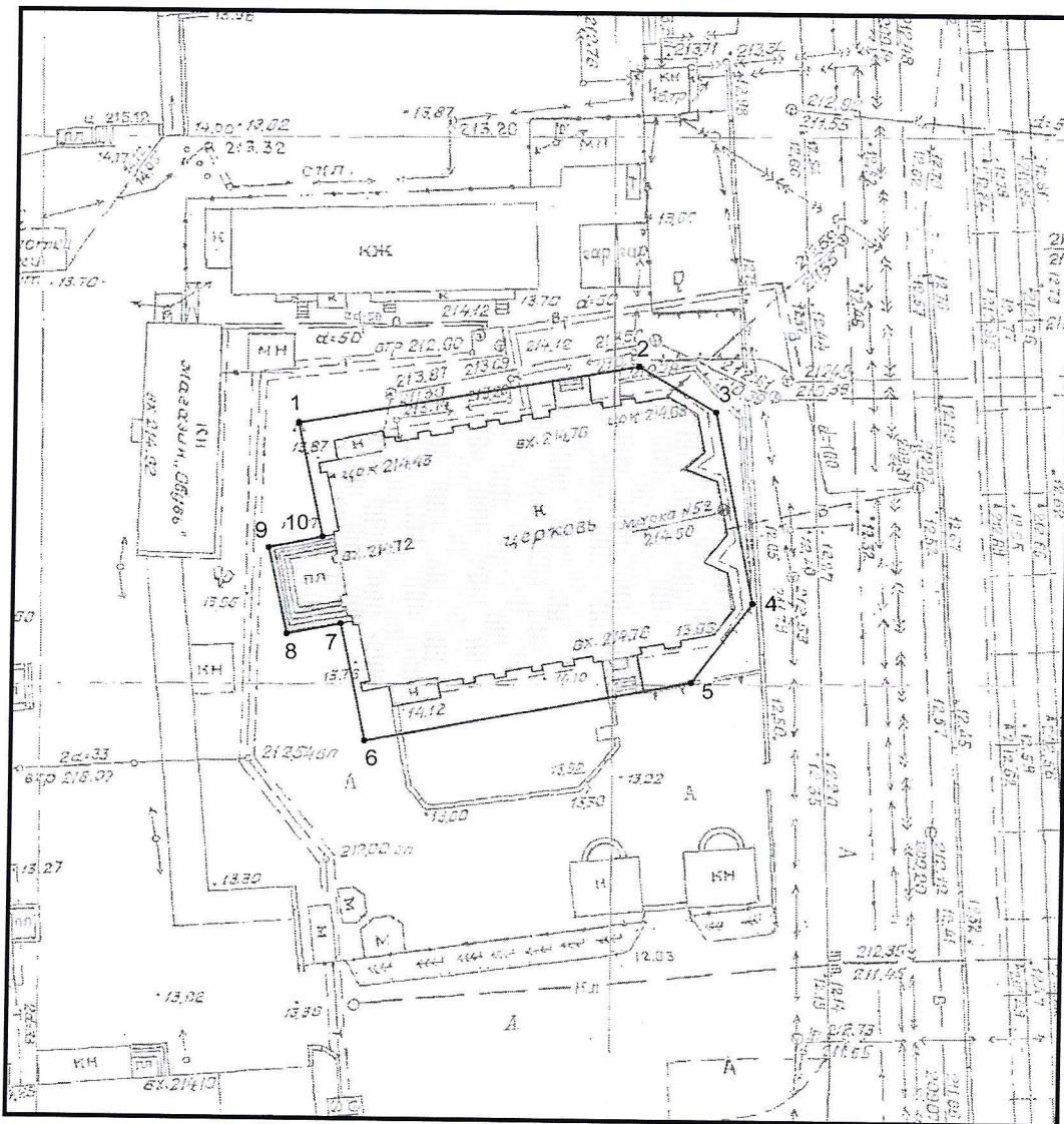
Условные обозначения к плану разбивки границ территории объекта культурного наследия регионального значения «Троицкая церковь»
