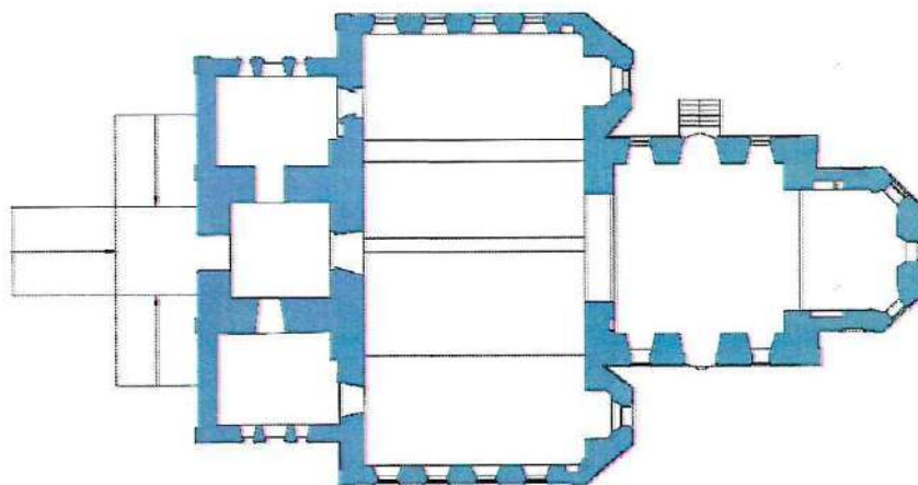
Рис. 3. План-схема первого этажа Объекта.
