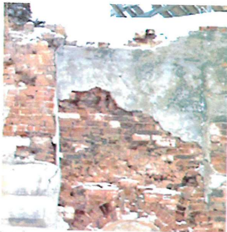
Рис. 14. Фотофиксация дефектов. Обрушение штукатурного слоя, структурное разрушение лицевой поверхности кладки стен, разрушение карнизной части стены.
