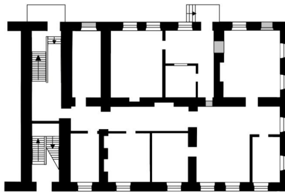
Рис. 11. Схема плана подвала.
