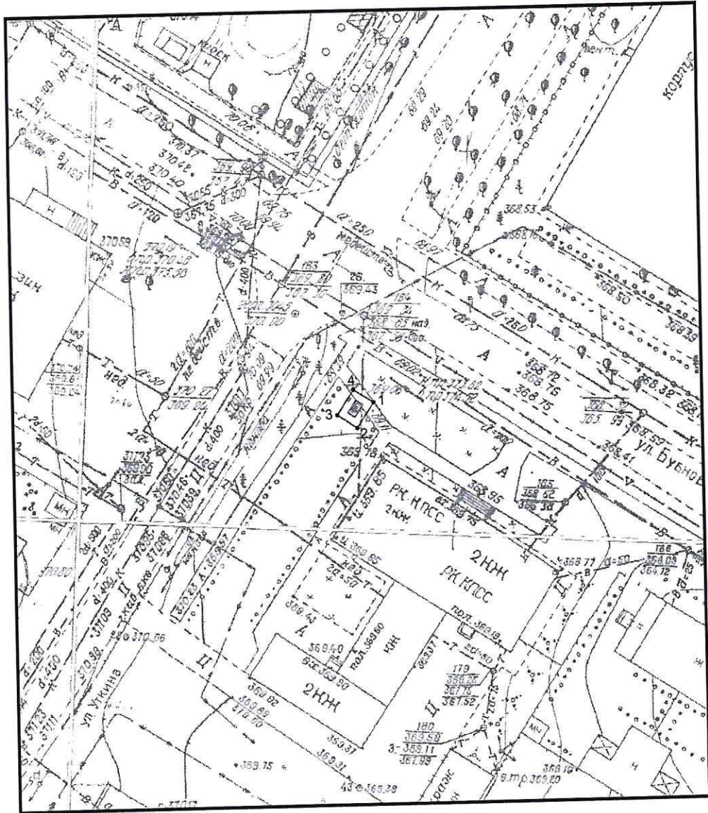
Условные обозначения к плану разбивки границ территории объекта культурного наследия регионального значения «Памятник В.И. Ленину»
