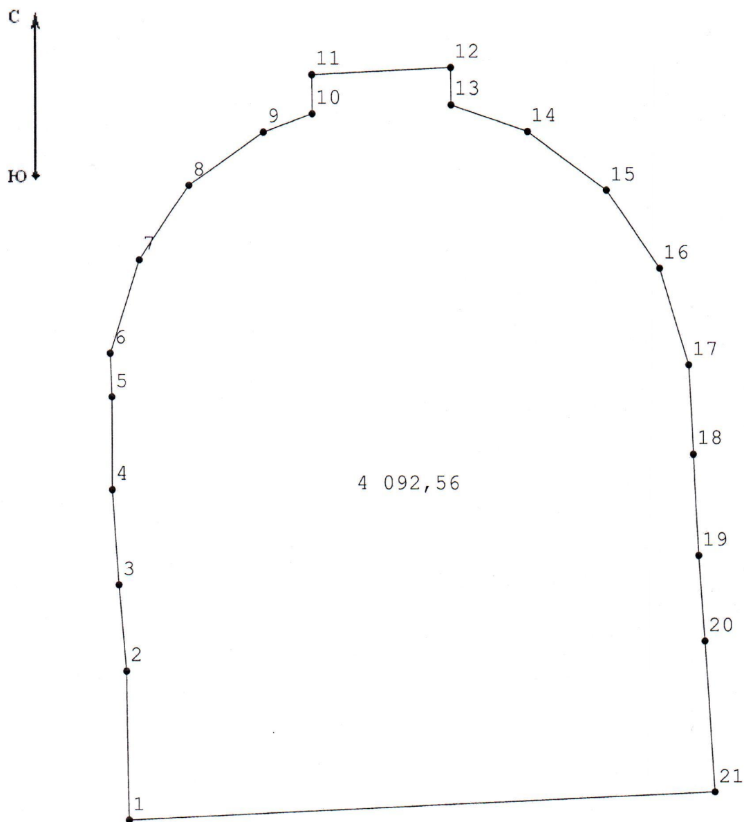
План границ
