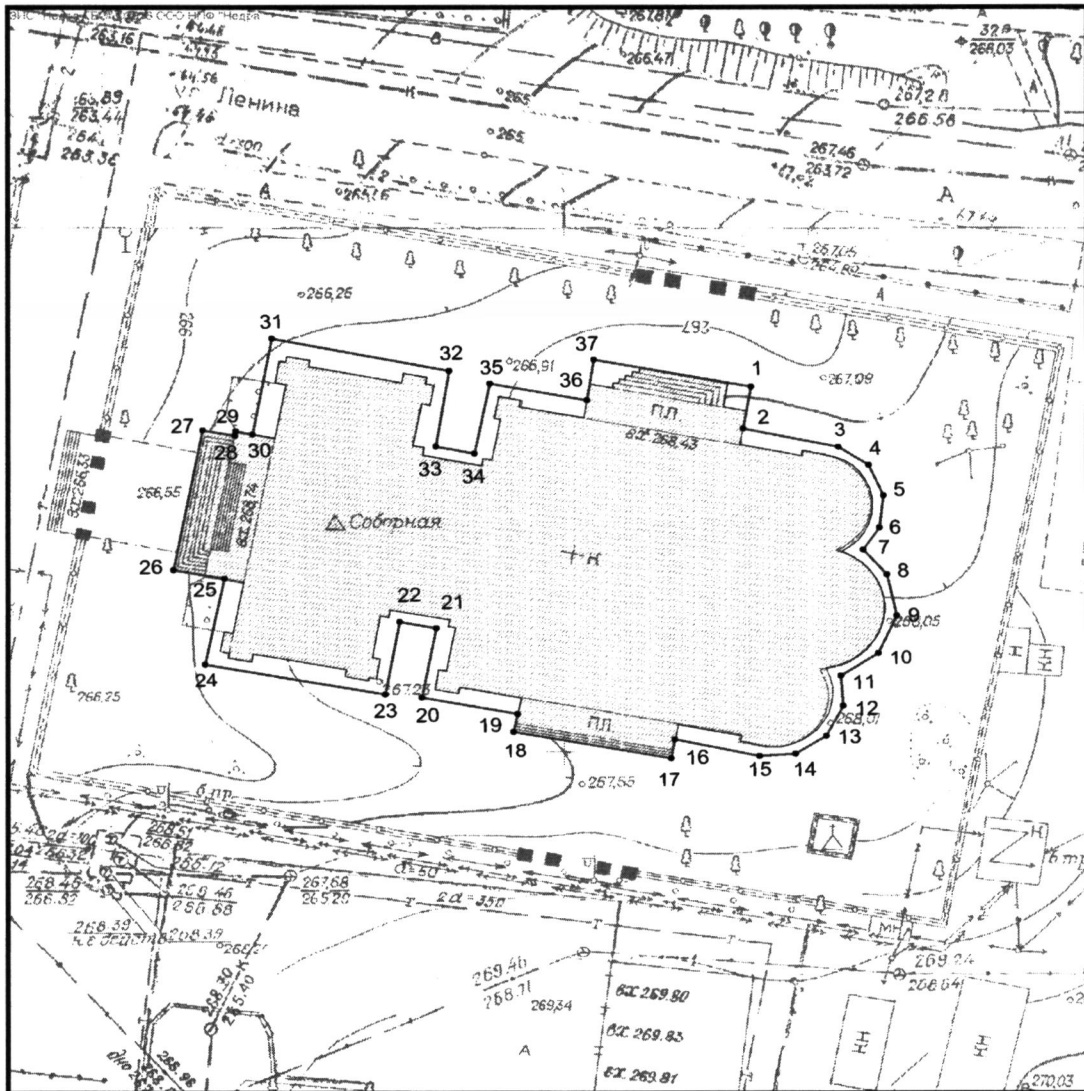
Условные обозначения к плану разбивки границ территории объекта культурного наследия регионального значения «Собор XIX в. на площади»
