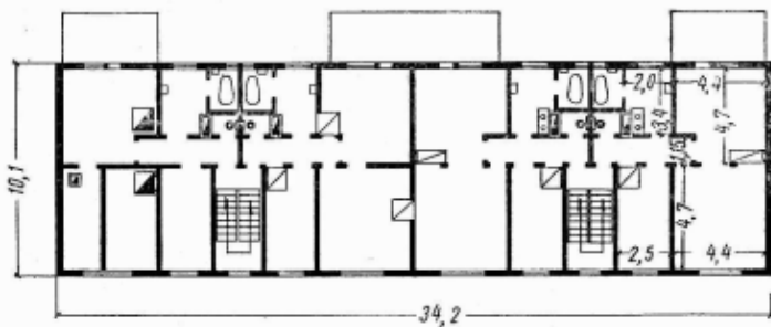
56. Жилые дома облегченной кон- струкции первых лет строительства Магнитогорска. План второго эта- жа и общий вид дома щитовой конструкции в «Березках»
