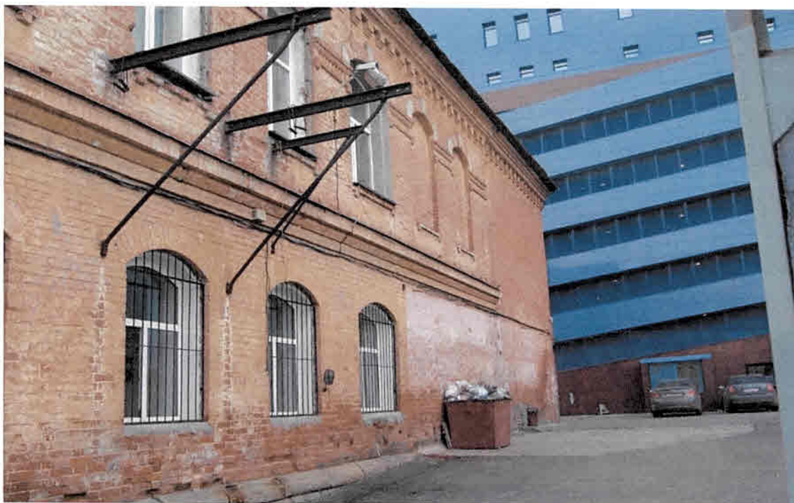
Фото 5. Фрагмент западного фасада здания
